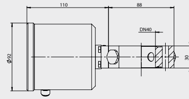
Raccord laitier DIN ITM-4DW/GG pour DN25...DN40
