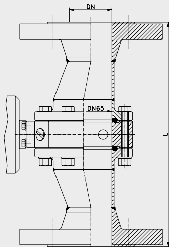
Bride DIN ITM-4DW/DF pour DN50...DN100
