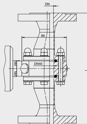
Bride DIN ITM-4DW/DF pour DN25...DN40
