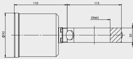
Raccord laitier DIN ITM-4DW/GG pour DN50...DN100
