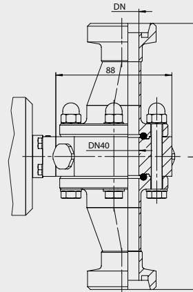
Raccord laitier DIN ITM-4DW/GG pour DN25...DN40
