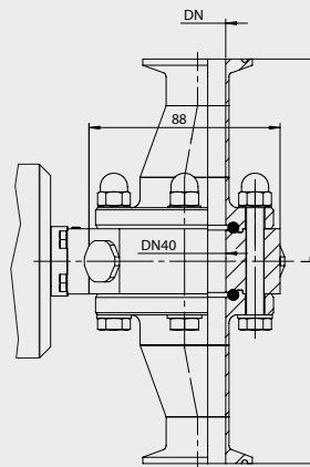
Tri-Clamp DIN ITM-4DW/TC pour DN25...DN40
