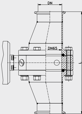
Tri-Clamp DIN ITM-4DW/TC pour DN50...DN100
