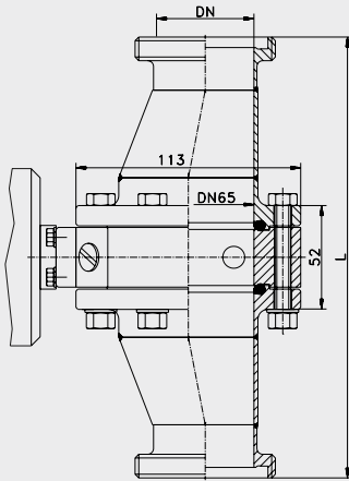
Raccord laitier DIN ITM-4DW/GG pour DN50...DN100
